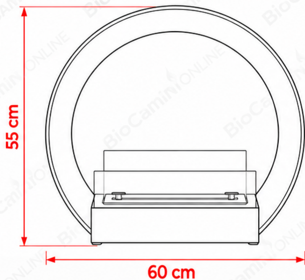
VISTA FRONTALE
