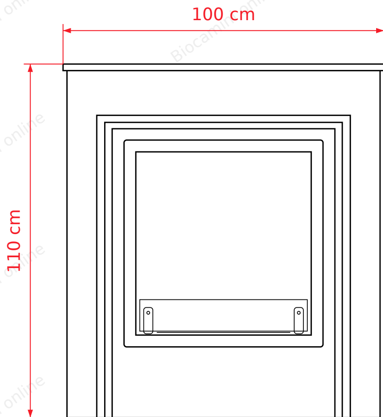
VISTA FRONTALE
