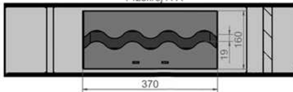
Przekrój A-A
