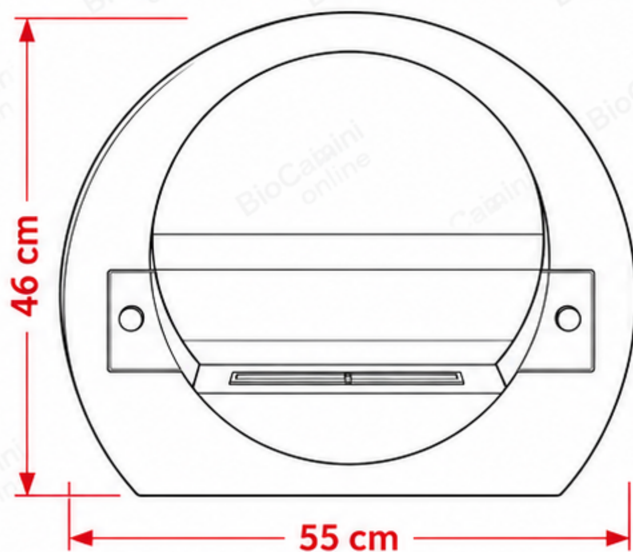
VISTA FRONTALE
