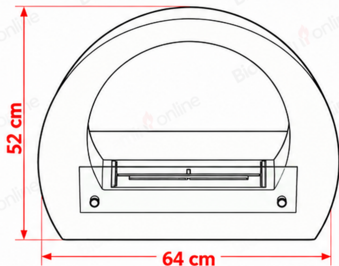
VISTA FRONTALE
