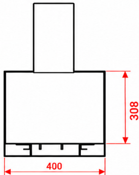
Przekrój B-B
