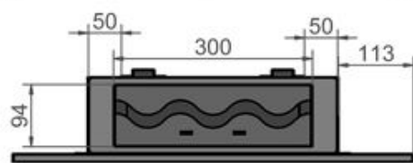
Przekrój A-A
