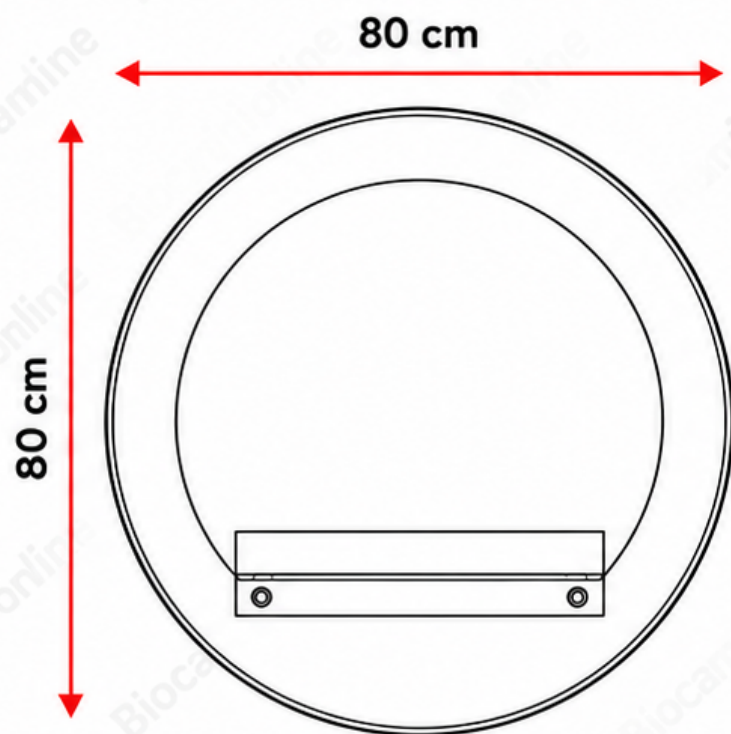
VISTA FRONTALE
