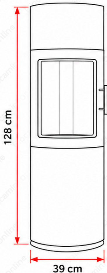
VISTA FRONTALE
