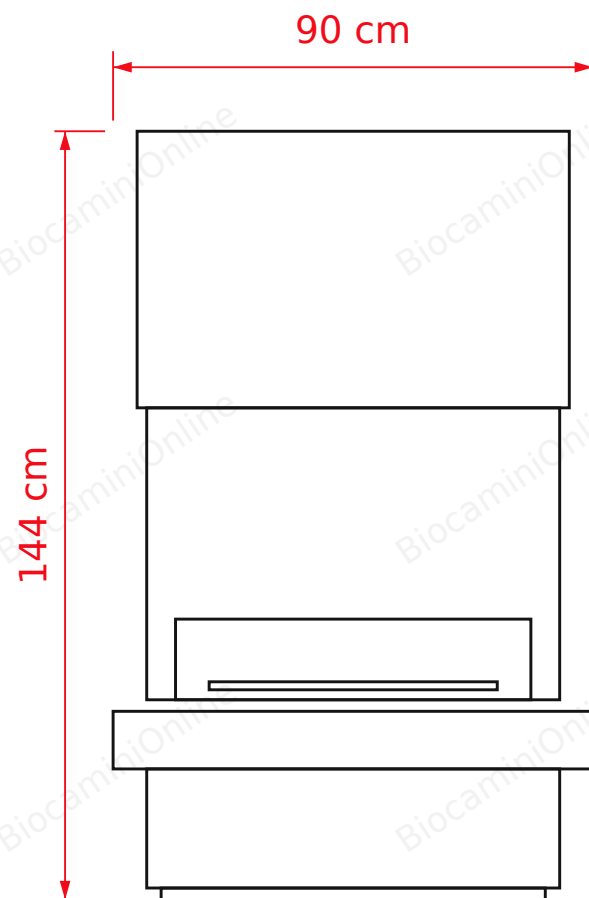
VISTA FRONTALE
