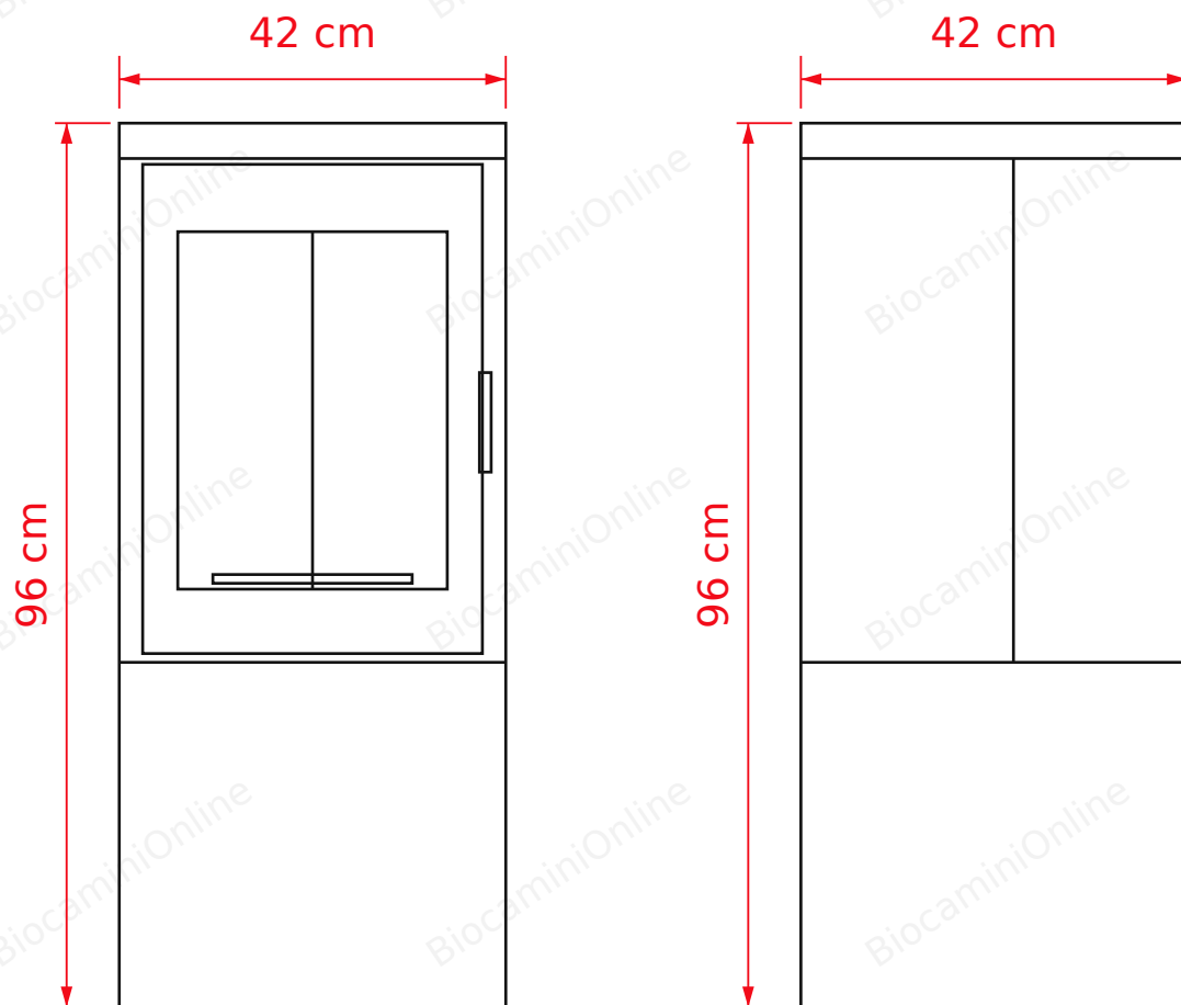
VISTA FRONTALE
