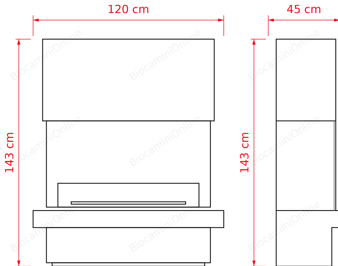
VISTA FRONTALE
